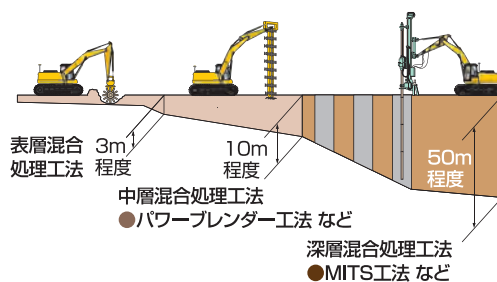
■各混合処理工法における施工深度の違い
