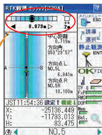
現況測量画面
