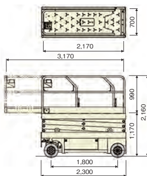
◎車両寸法図 (ENTL080)
