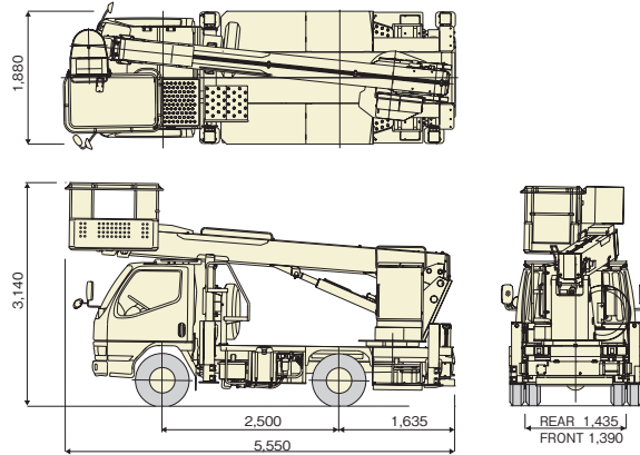
◎車両寸法図 (AT-130TG)
