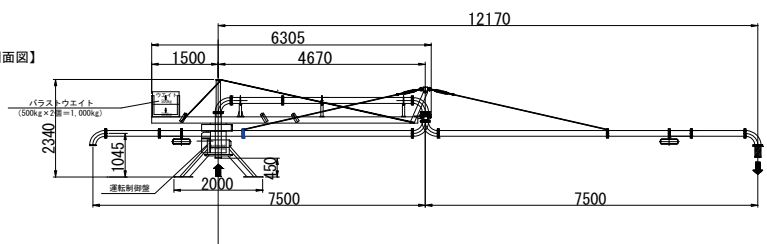
【正面図】
